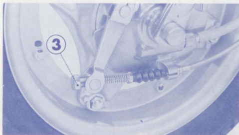
③ Einstellmutter der Vorderradbremse
