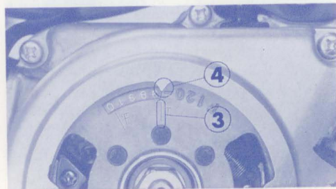
③ "F"-Marke ④ Einstellmarke
