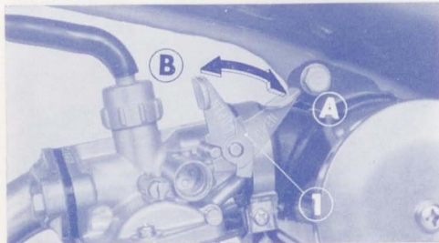
① Starterklappenhebel
