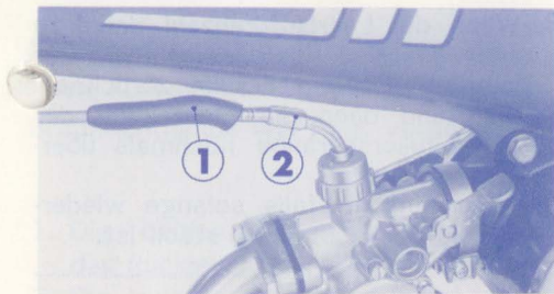
① Gummiüberzug ② Gaszugeinsteller
