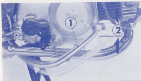
① Fußbremshebel ② Spiel
