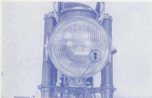
① Befestigungsschraube des Scheinwerferrings
