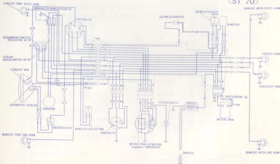
LICHTSCHALTER SCHALTBILD
