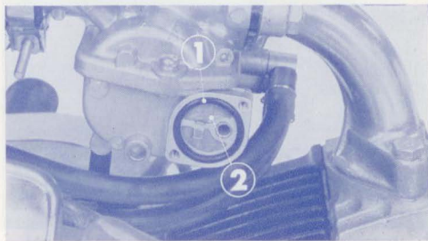
① O-Ringdichtung ② Kraftstoffsieb
