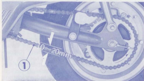
① Antriebskette
